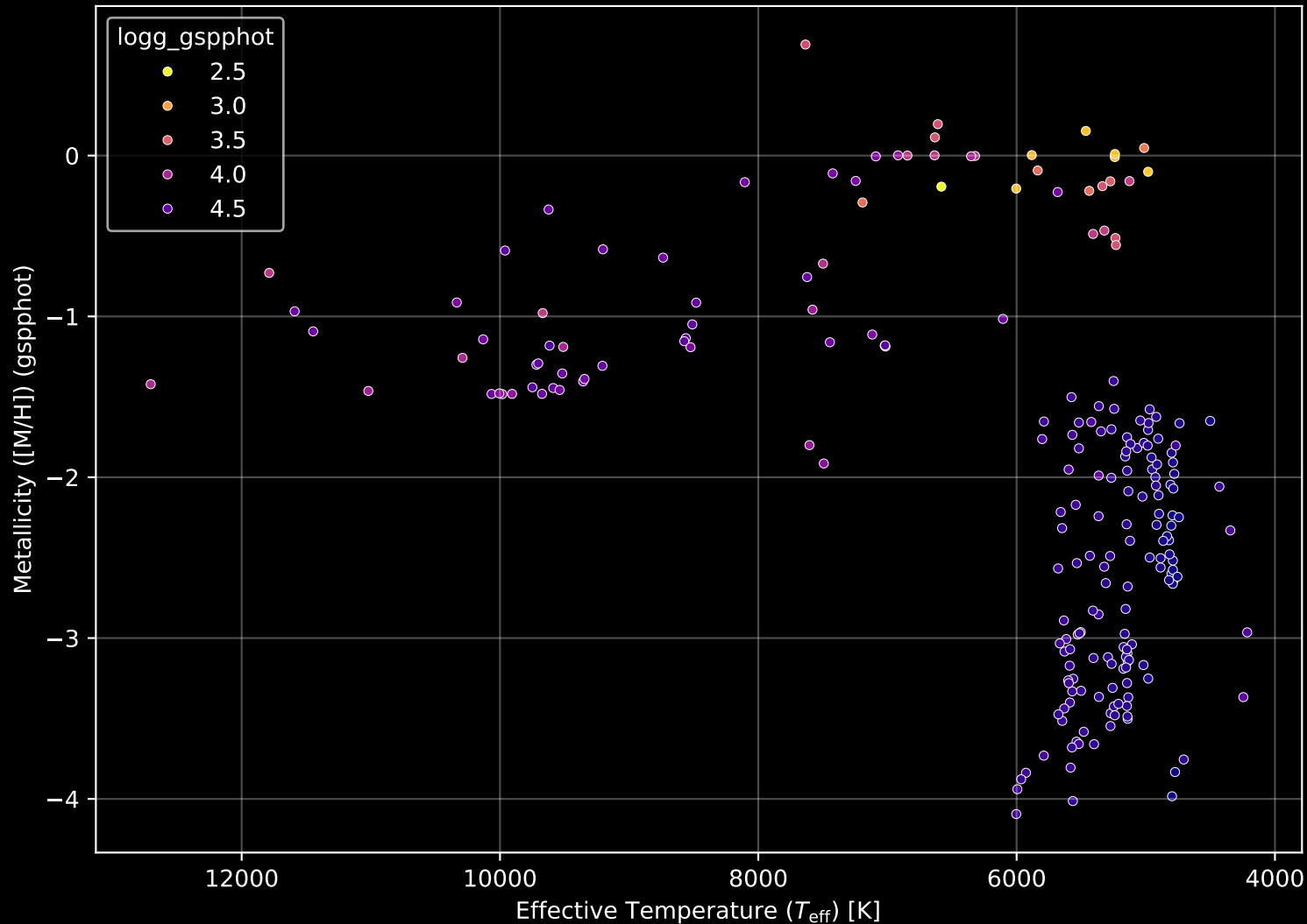
Gaia Cluster: [Berkeley_76] Stellar Population Parameters (n= 220)
