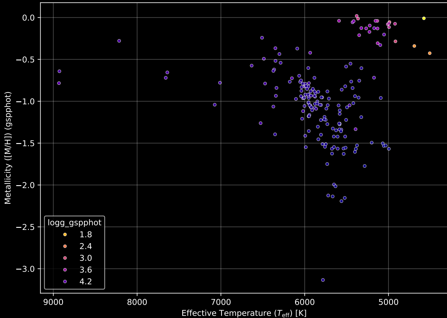
Gaia Cluster: [Berkeley_78] Stellar Population Parameters (n= 182)
