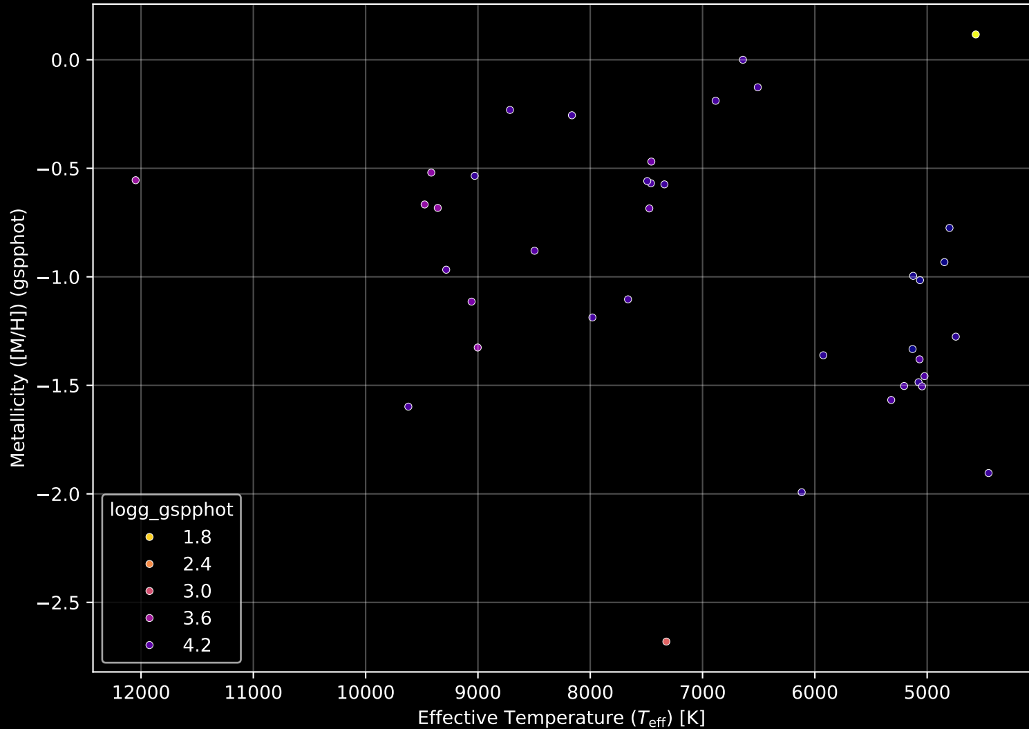
Gaia Cluster: [Berkeley_82] Stellar Population Parameters (n= 39)
