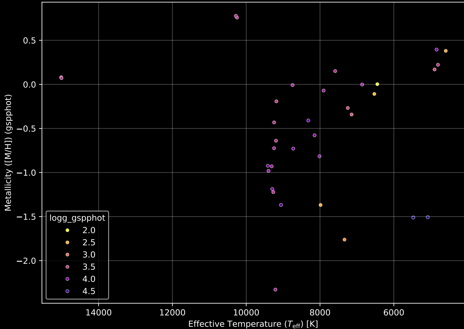
Gaia Cluster: [Berkeley_83] Stellar Population Parameters (n= 35)
