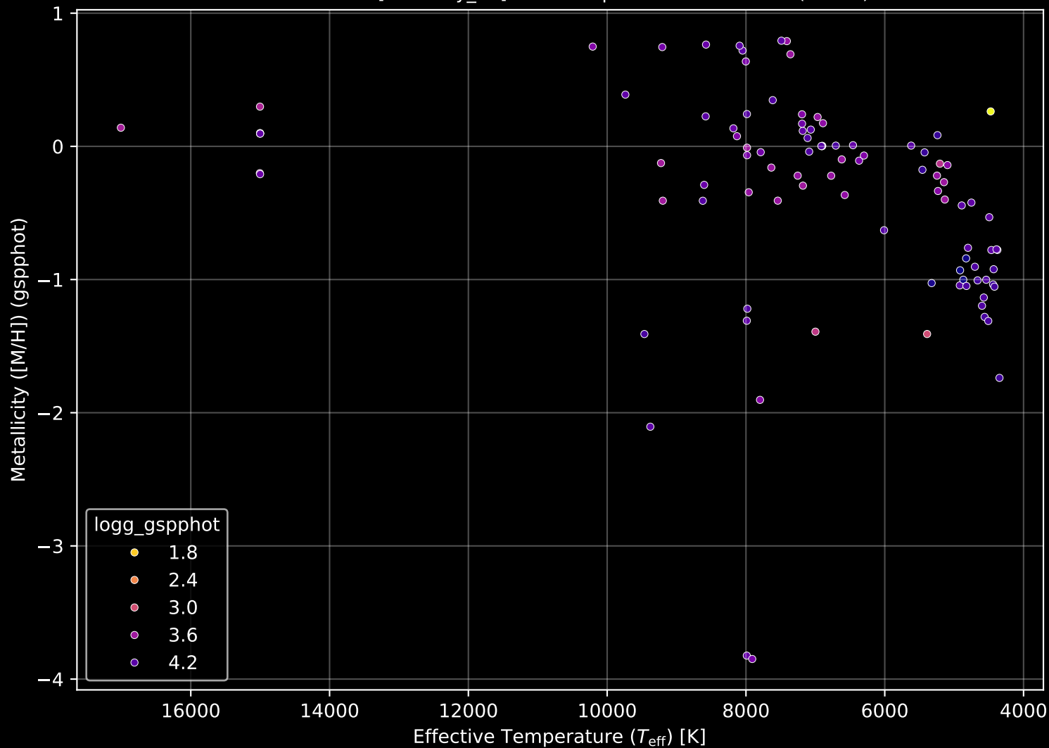
Gaia Cluster: [Berkeley_86] Stellar Population Parameters (n= 98)
