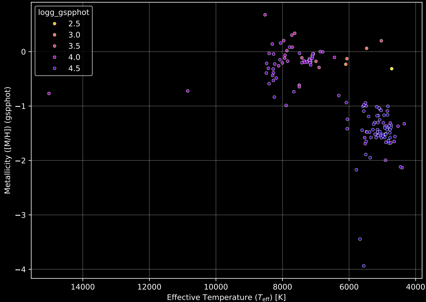
Gaia Cluster: [Berkeley_9] Stellar Population Parameters (n= 141)
