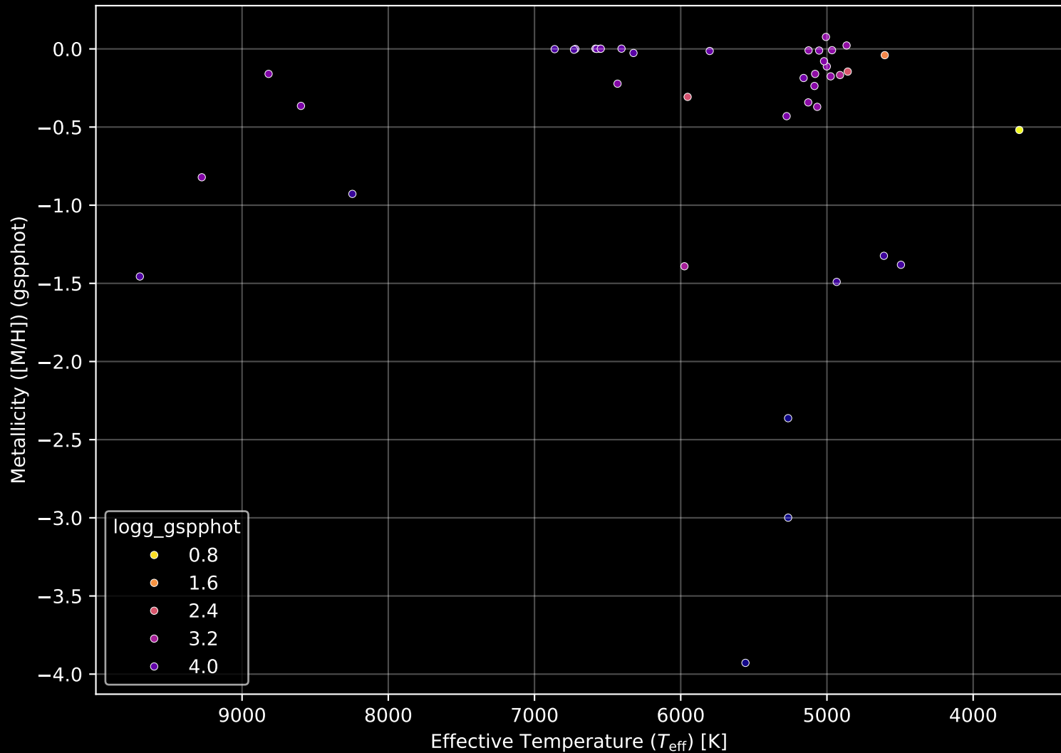
Gaia Cluster: [Berkeley_92] Stellar Population Parameters (n= 42)
