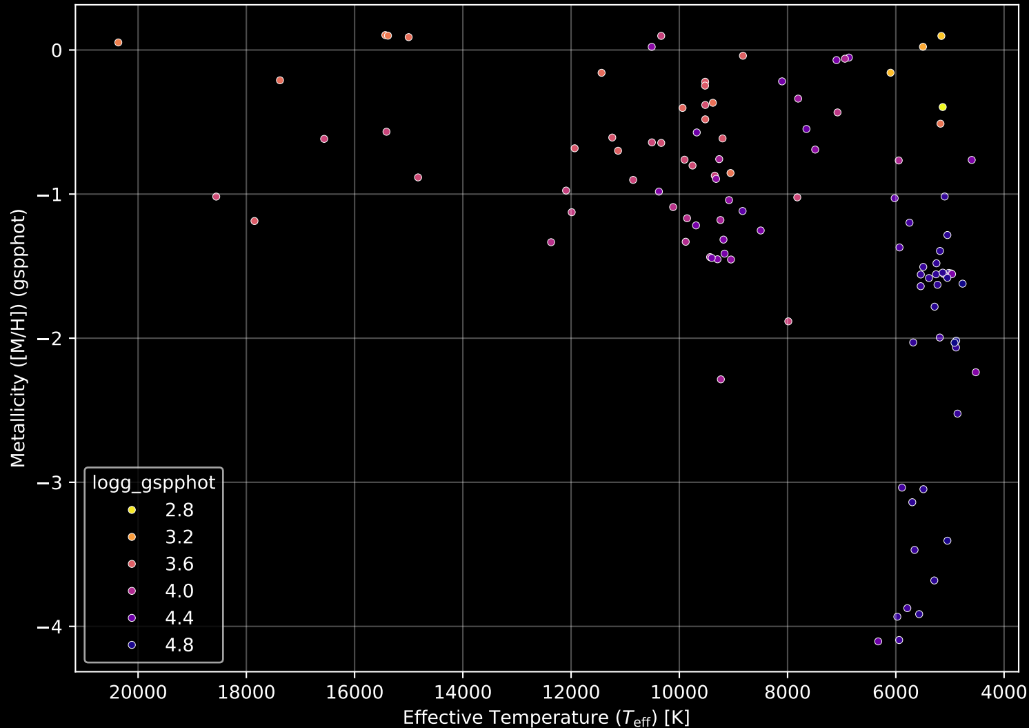
Gaia Cluster: [Berkeley_94] Stellar Population Parameters (n= 109)
