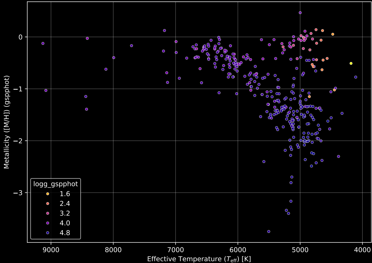
Gaia Cluster: [Berkeley_98] Stellar Population Parameters (n= 328)
