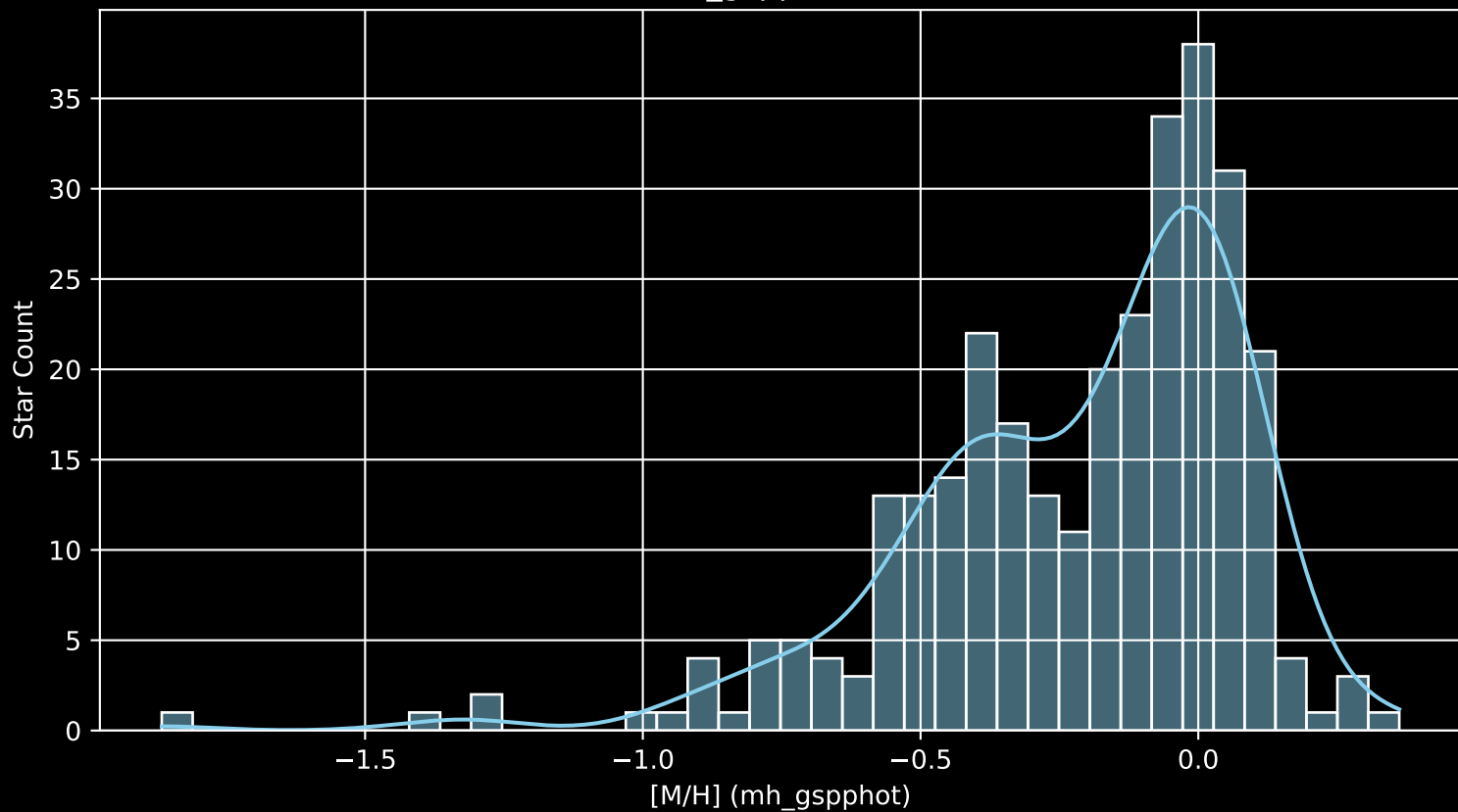
Gaia Cluster: [Blanco_1 [M/H] (mh_gspphot) (n= 307)
