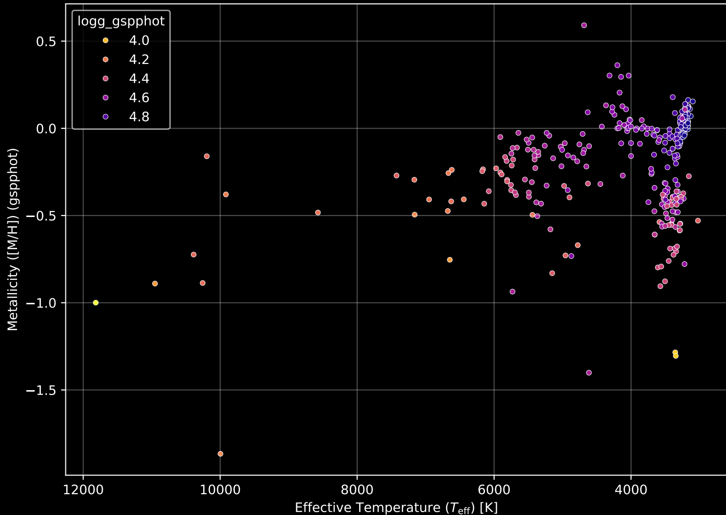
Gaia Cluster: [Blanco_1] Stellar Population Parameters (n= 308)
