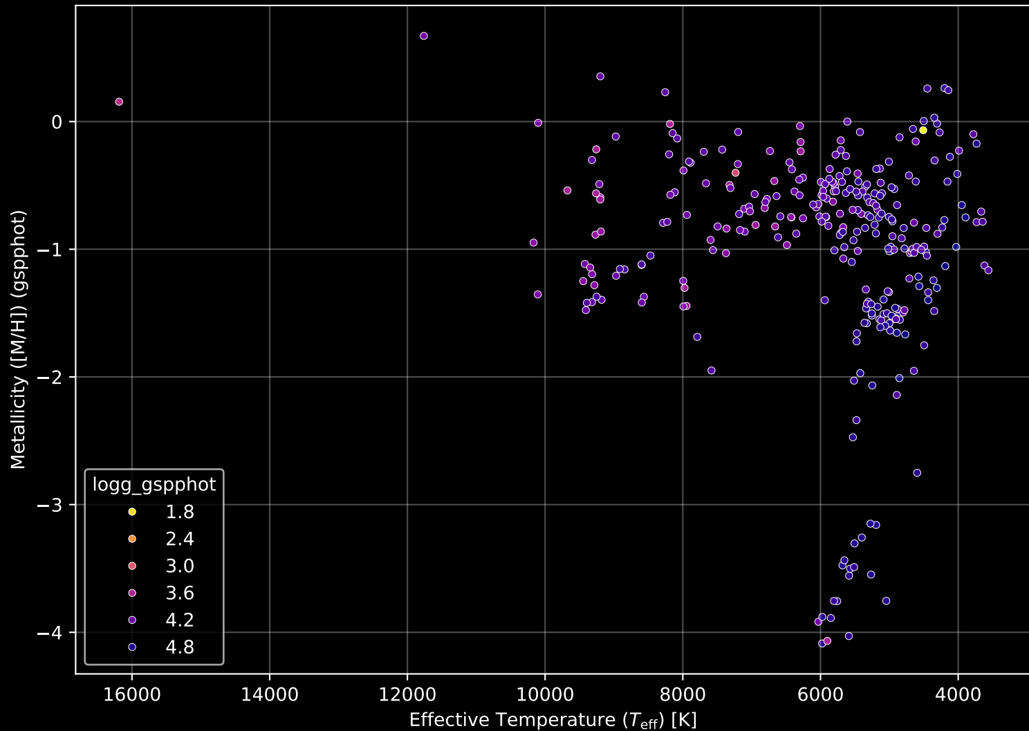
Gaia Cluster: [COIN-Gaia_23] Stellar Population Parameters (n= 302)
