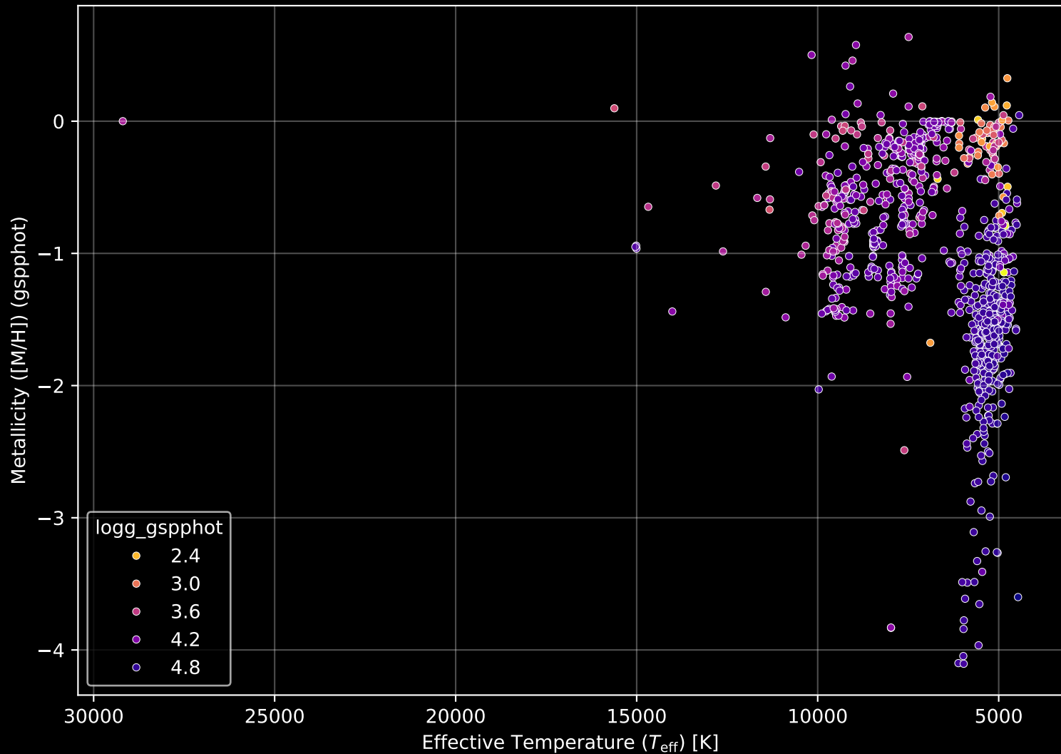
Gaia Cluster: [COIN-Gaia_4] Stellar Population Parameters (n= 1005)
