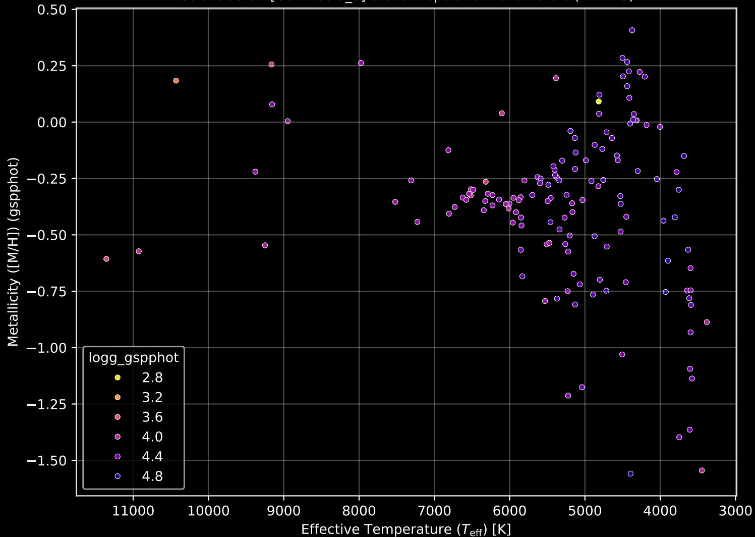
Gaia Cluster: [COIN-Gaia_8] Stellar Population Parameters (n= 143)
