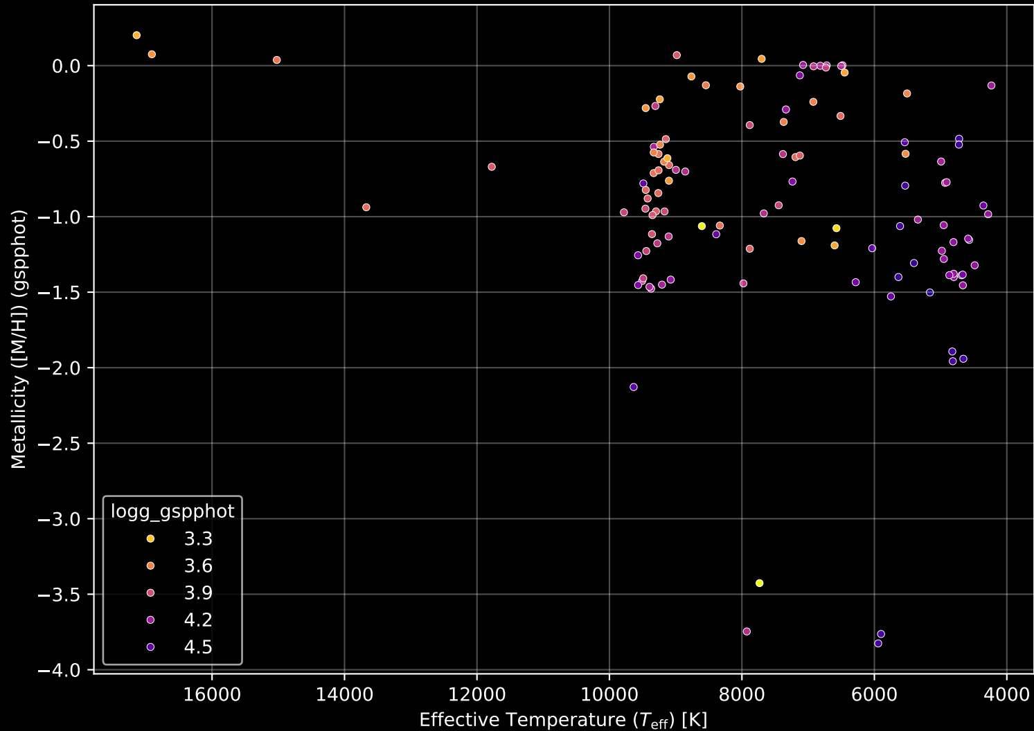
Gaia Cluster: [Collinder_205] Stellar Population Parameters (n= 116)
