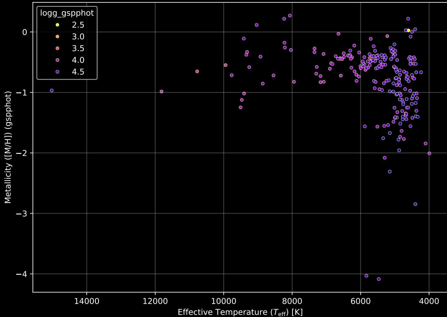
Gaia Cluster: [Collinder_258] Stellar Population Parameters (n= 217)
