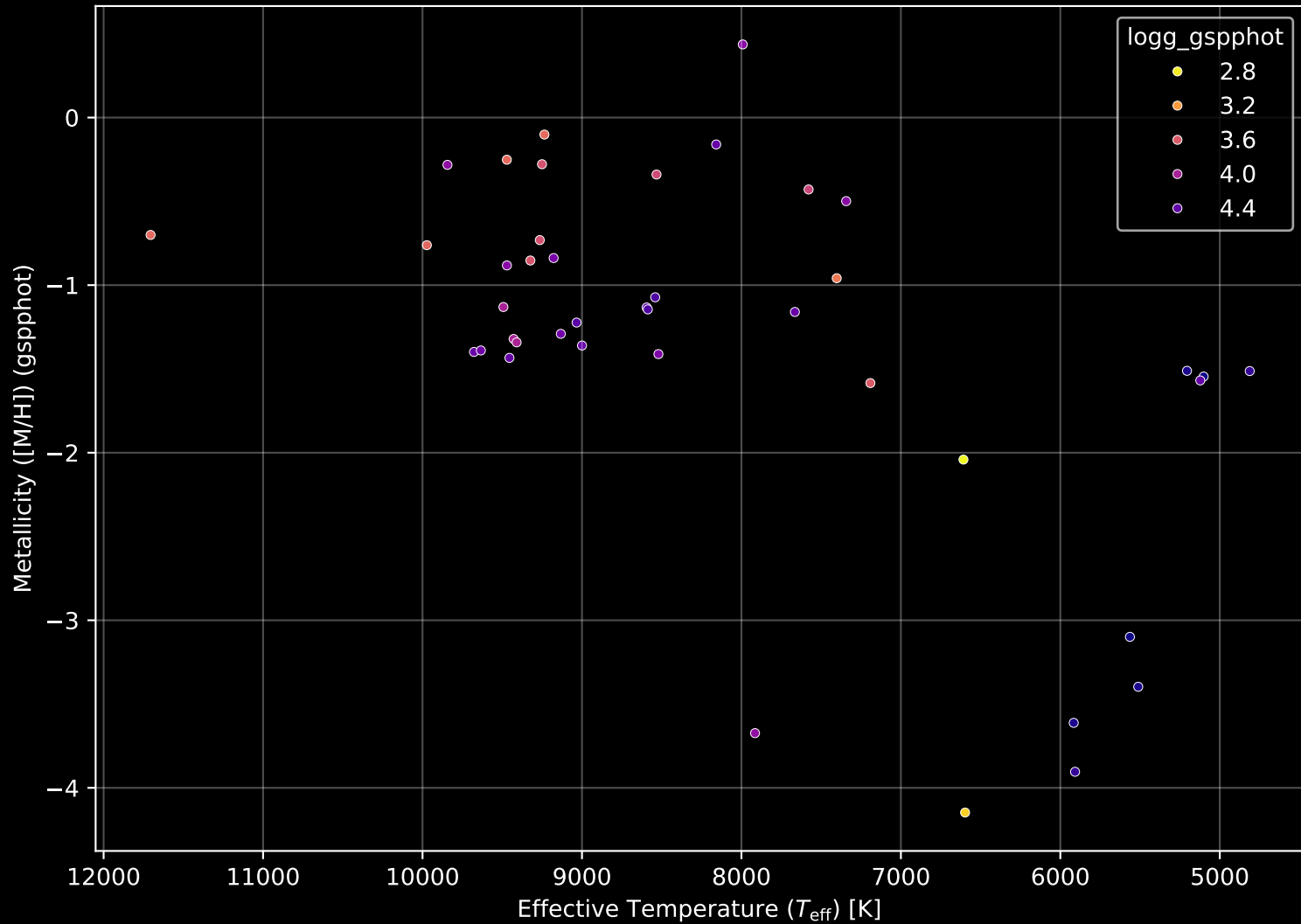
Gaia Cluster: [Czernik_1] Stellar Population Parameters (n= 42)
