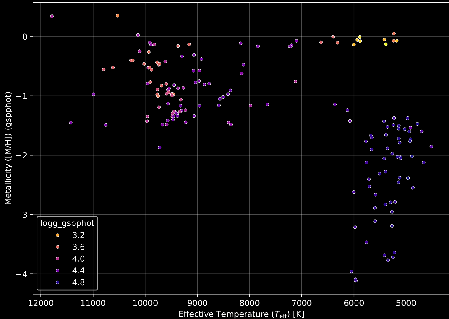
Gaia Cluster: [Czernik_13] Stellar Population Parameters (n= 168)
