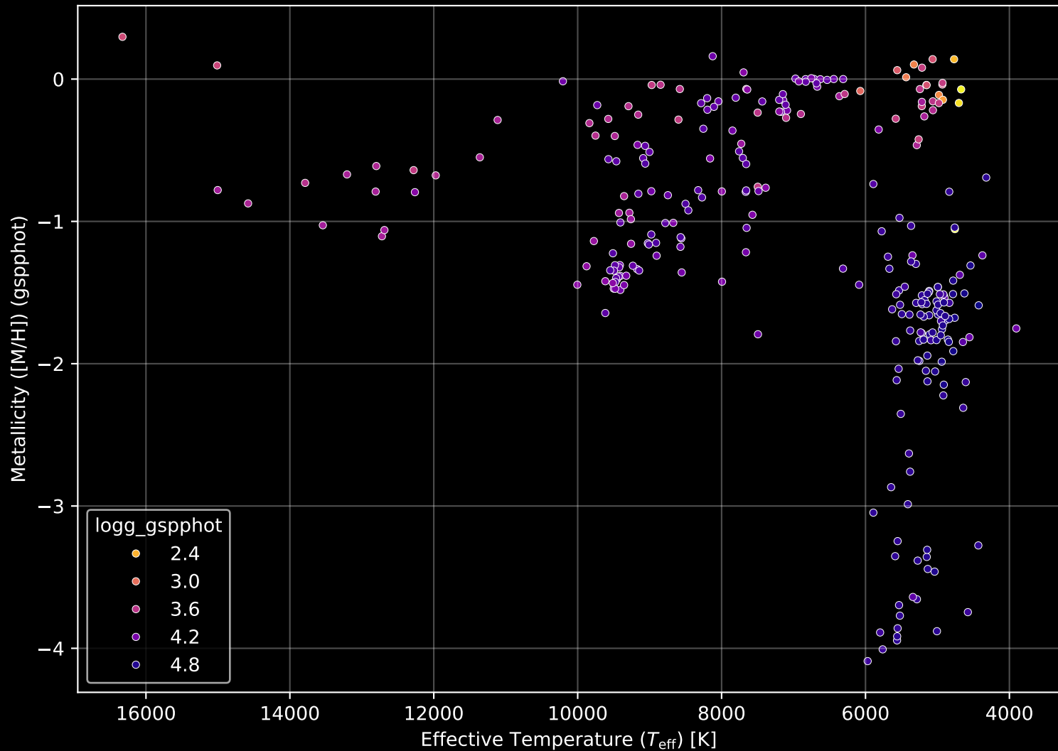
Gaia Cluster: [Czernik_15] Stellar Population Parameters (n= 281)
