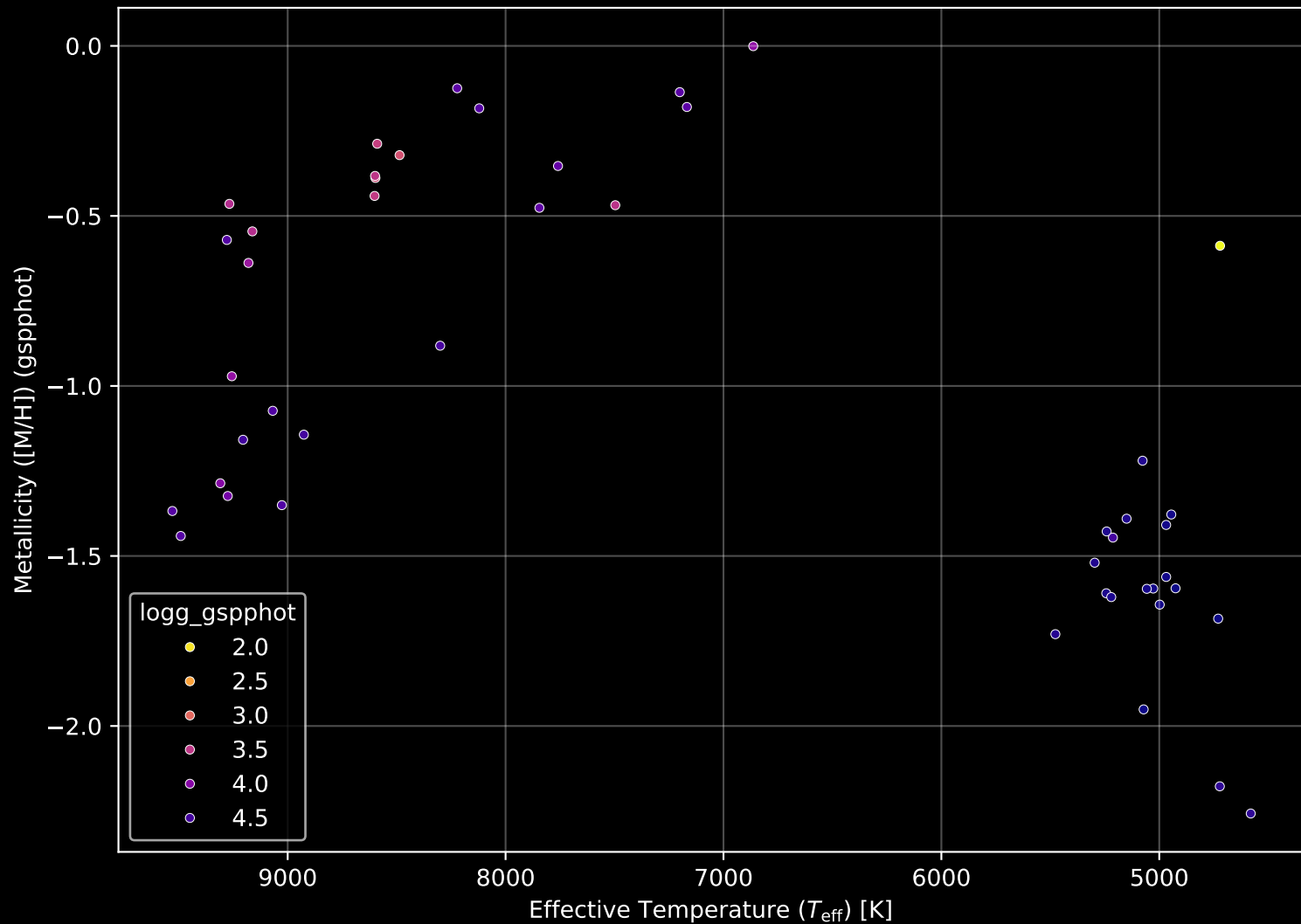
Gaia Cluster: [Czernik_16] Stellar Population Parameters (n= 47)
