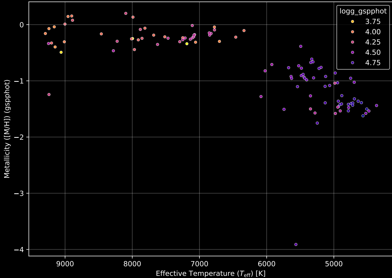
Gaia Cluster: [Czernik_2] Stellar Population Parameters (n= 108)
