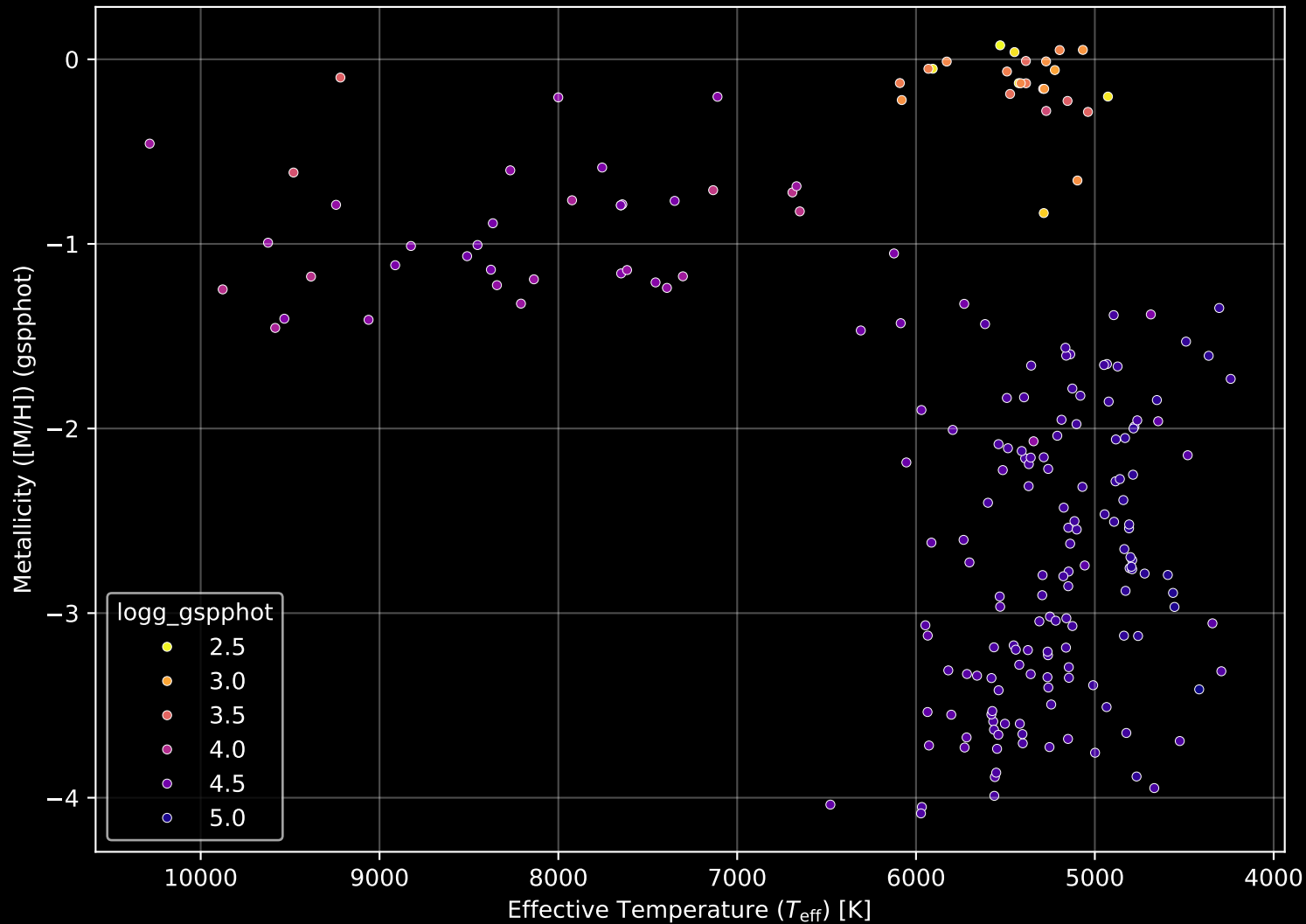
Gaia Cluster: [Czernik_24] Stellar Population Parameters (n= 208)
