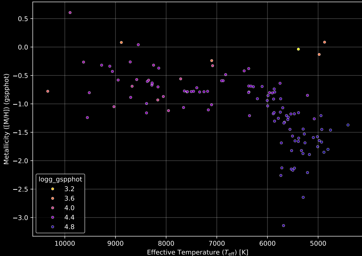
Gaia Cluster: [Czernik_27] Stellar Population Parameters (n= 118)
