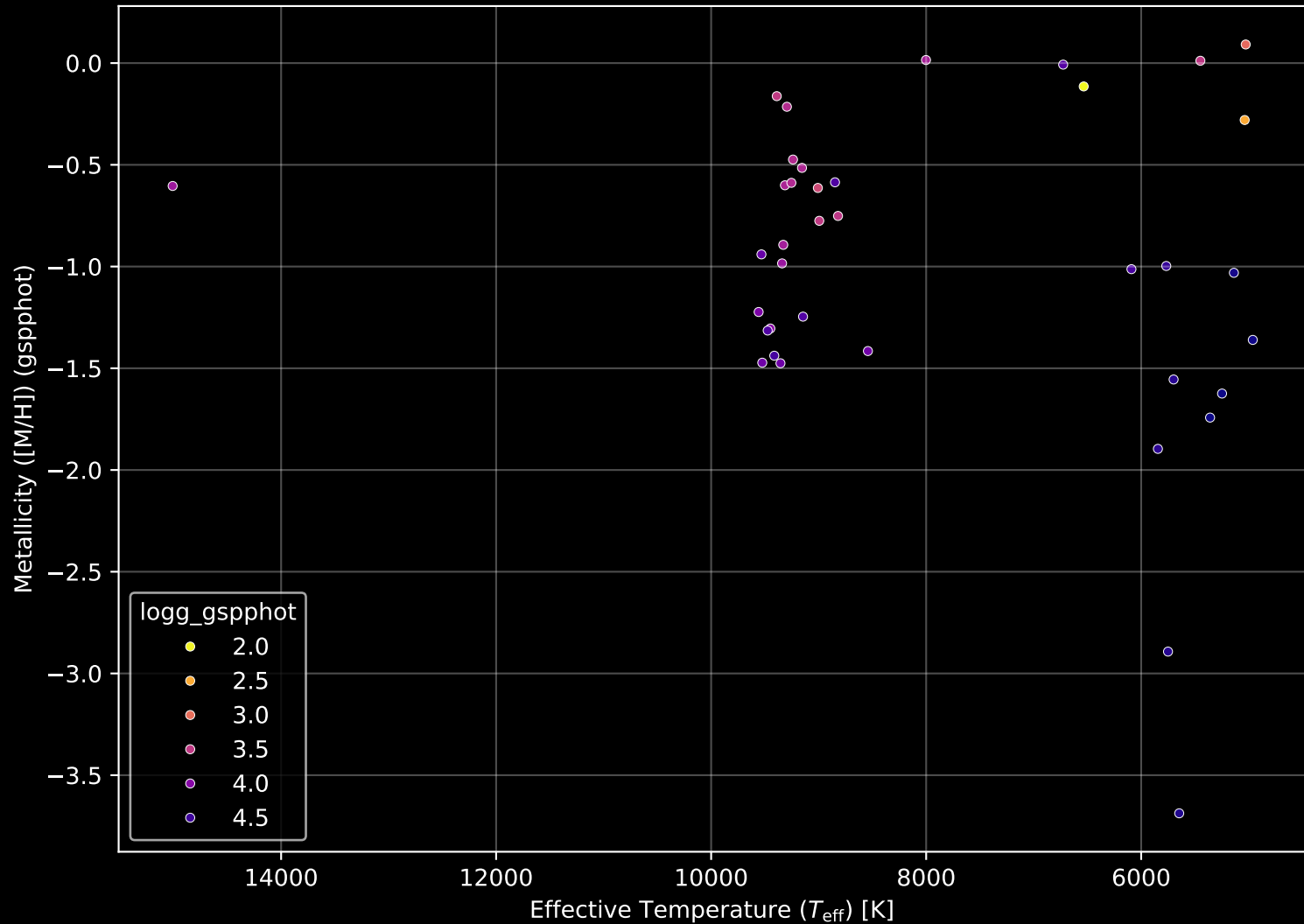
Gaia Cluster: [Czernik_3] Stellar Population Parameters (n= 38)
