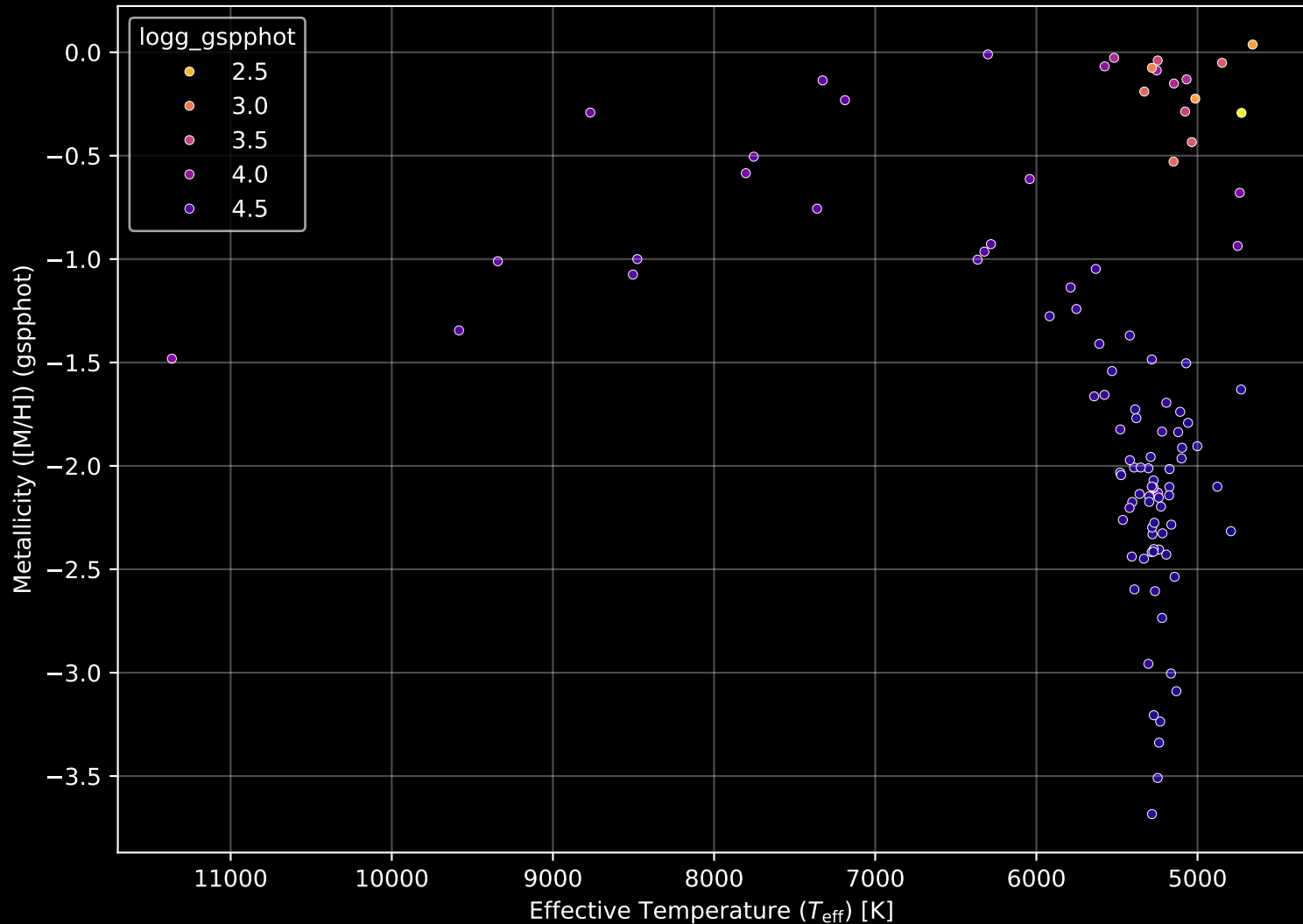
Gaia Cluster: [Czernik_30] Stellar Population Parameters (n= 105)
