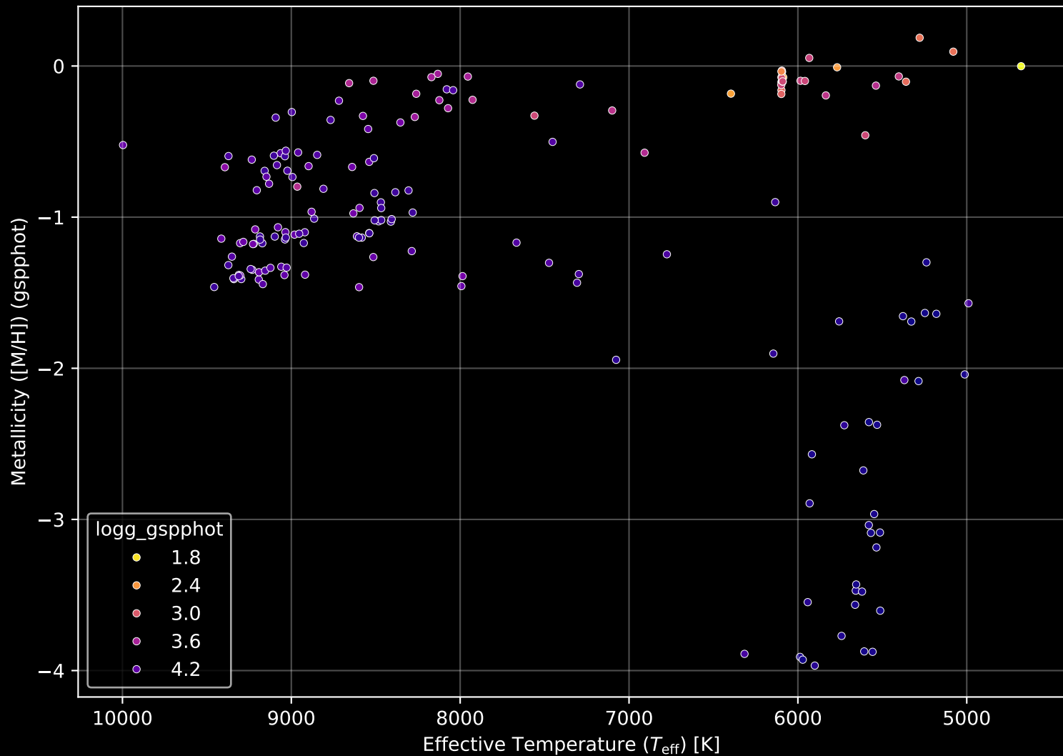
Gaia Cluster: [Czernik_32] Stellar Population Parameters (n= 181)
