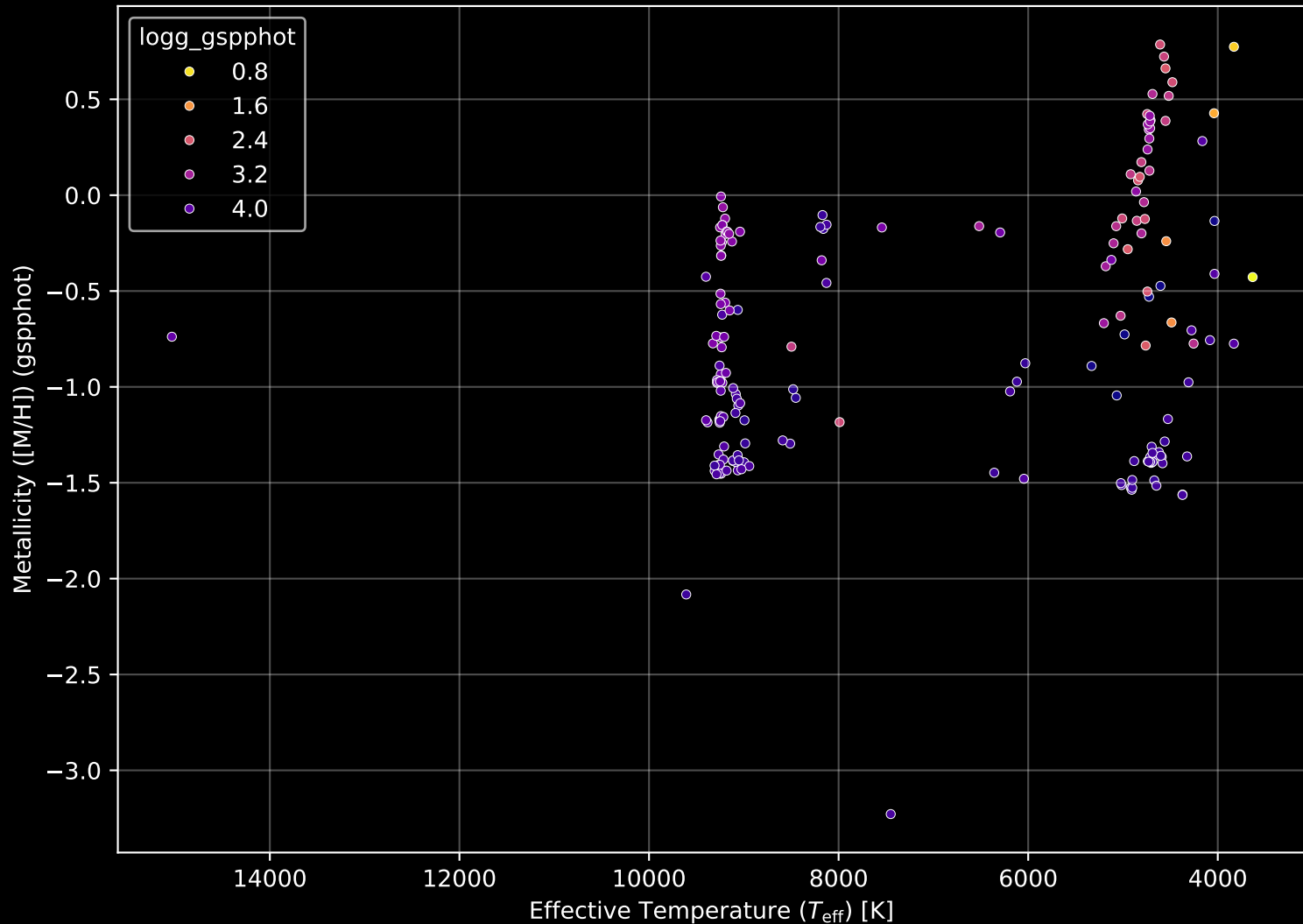
Gaia Cluster: [Czernik_38] Stellar Population Parameters (n= 186)
