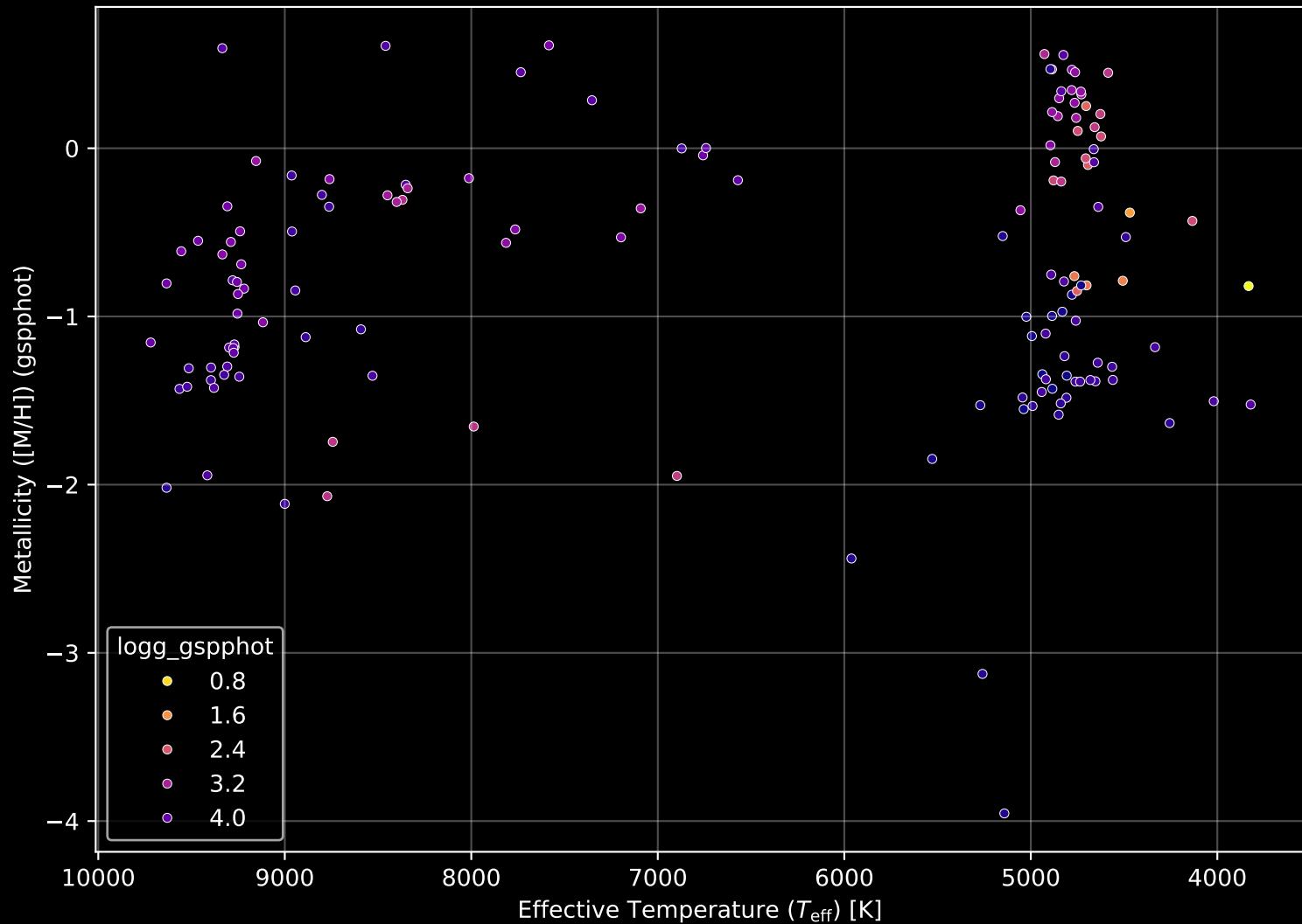
Gaia Cluster: [Czernik_39] Stellar Population Parameters (n= 143)
