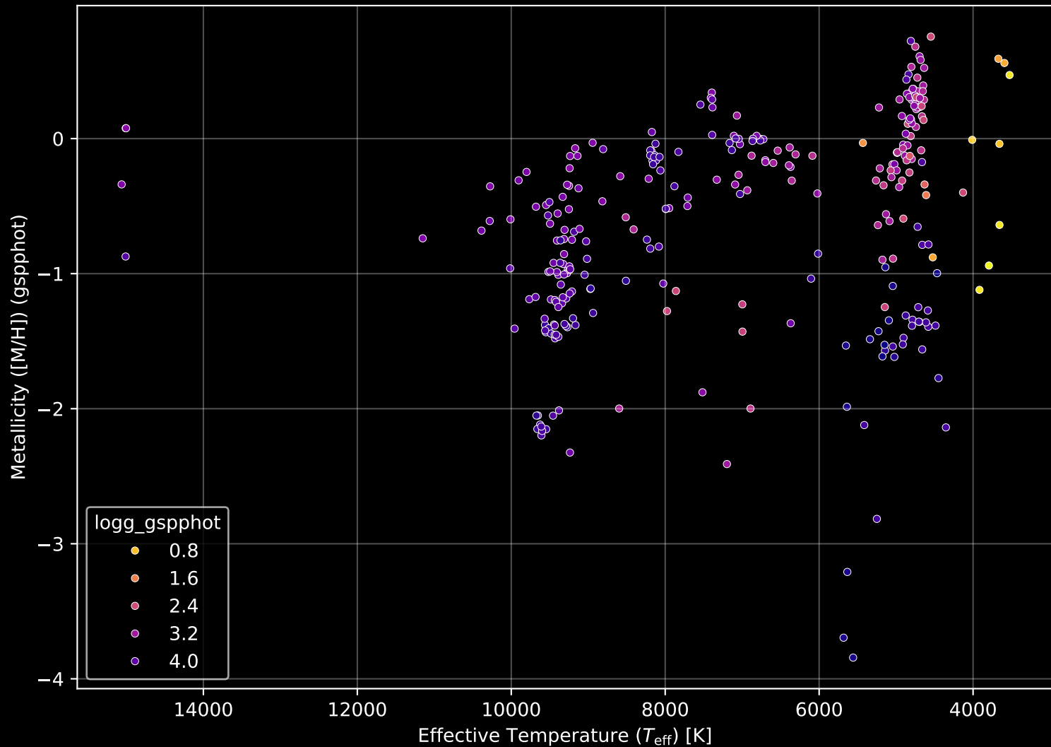
Gaia Cluster: [Czernik_40] Stellar Population Parameters (n= 304)
