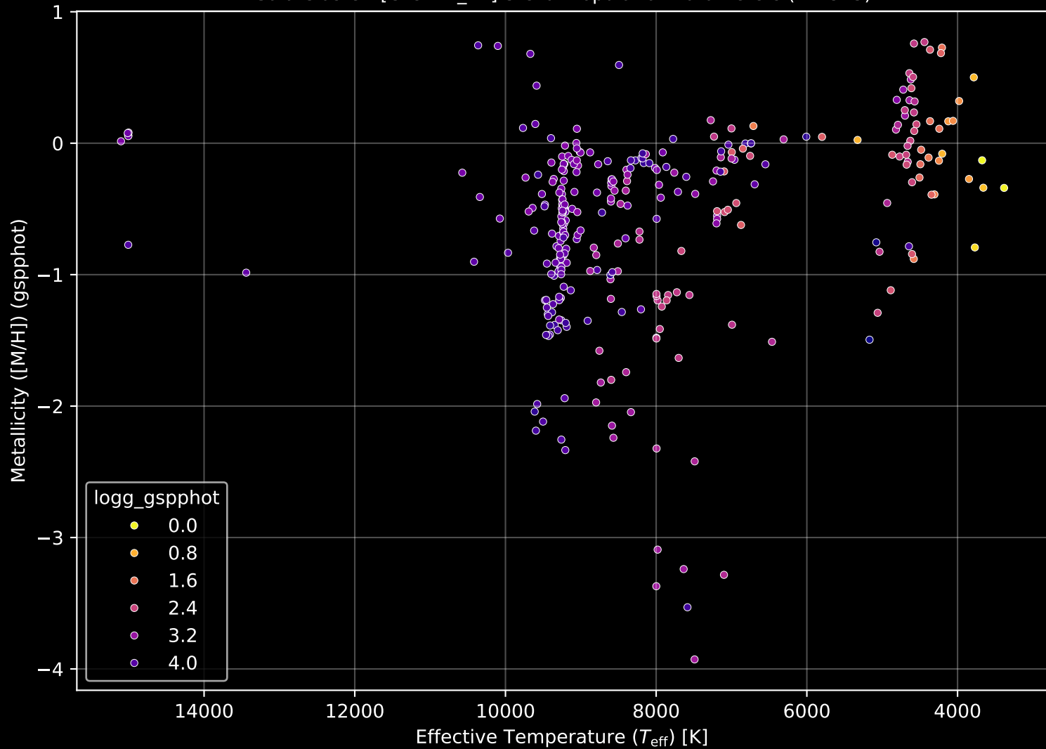
Gaia Cluster: [Czernik_41] Stellar Population Parameters (n= 315)
