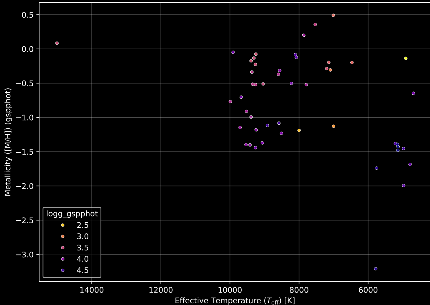
Gaia Cluster: [Czernik_42] Stellar Population Parameters (n= 49)
