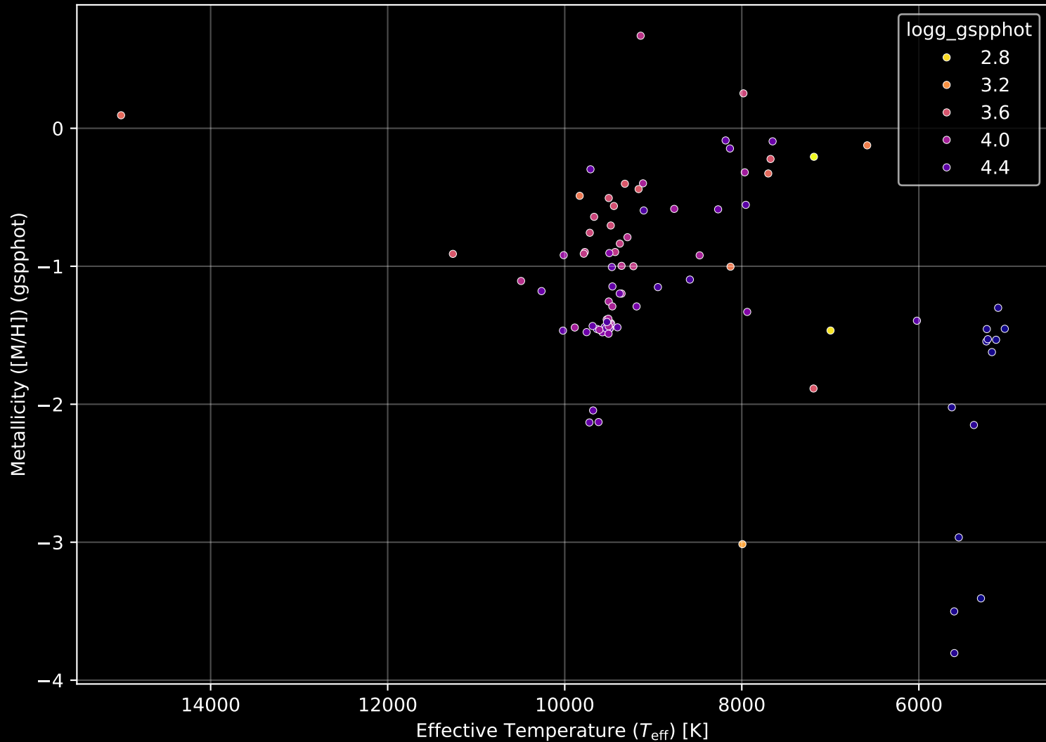
Gaia Cluster: [Czernik_44] Stellar Population Parameters (n= 93)
