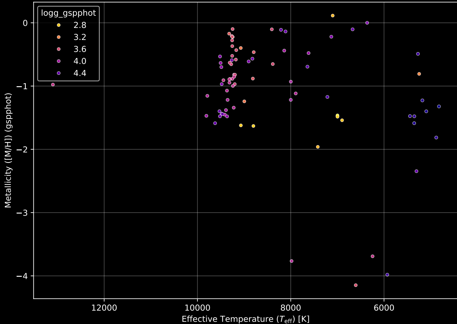
Gaia Cluster: [Czernik_5] Stellar Population Parameters (n= 83)
