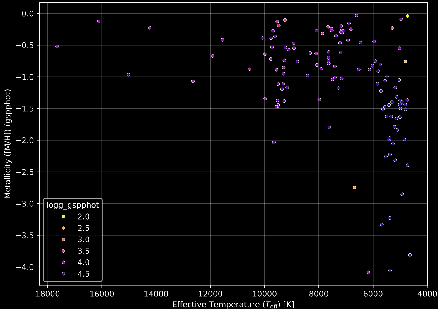
Gaia Cluster: [Czernik_6] Stellar Population Parameters (n= 125)
