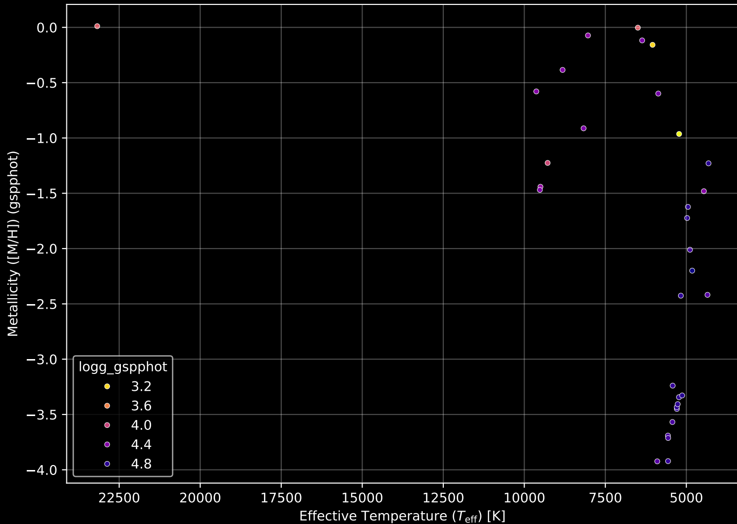
Gaia Cluster: [DC_8] Stellar Population Parameters (n= 32)
