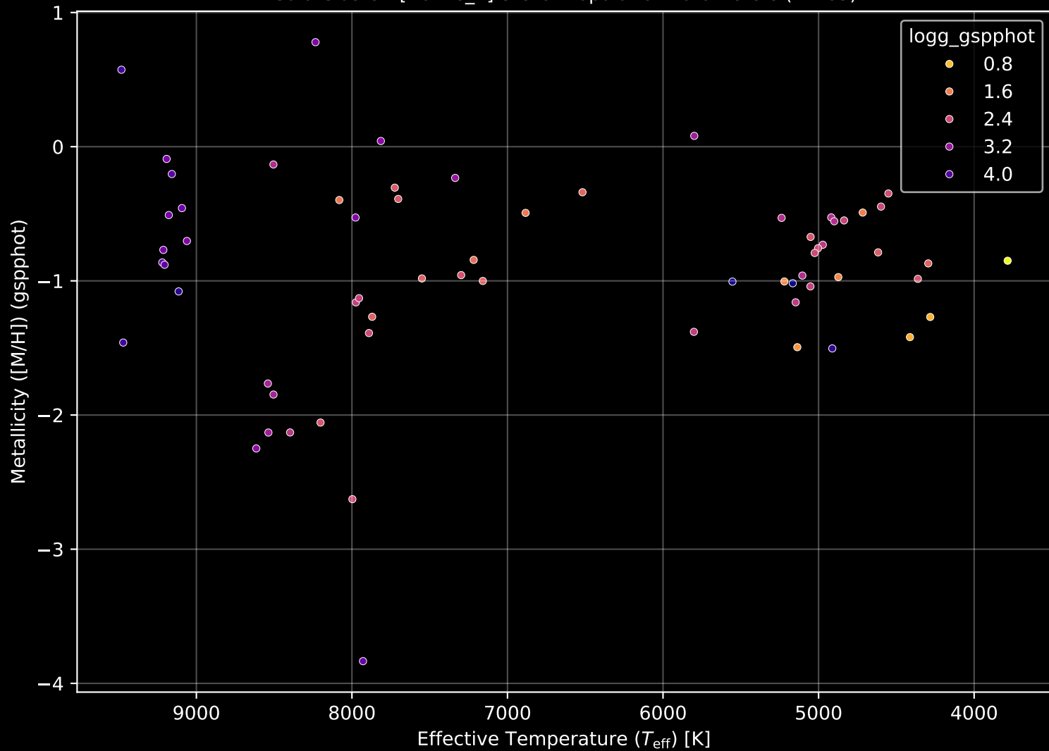
Gaia Cluster: [Danks_1] Stellar Population Parameters (n= 65)
