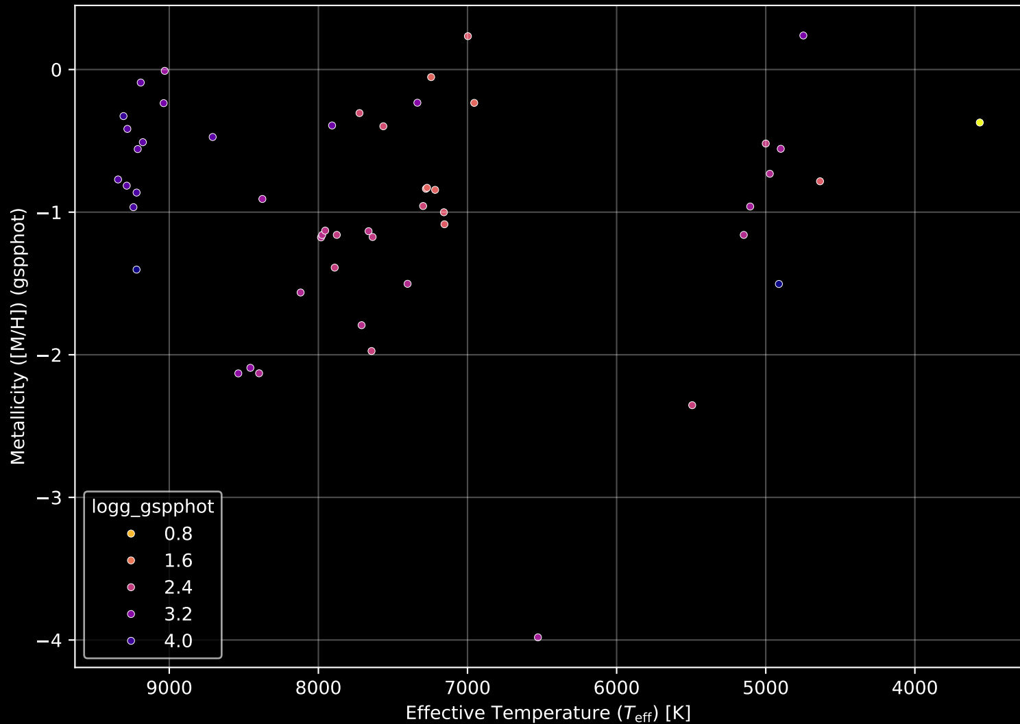
Gaia Cluster: [Danks_2] Stellar Population Parameters (n= 52)
