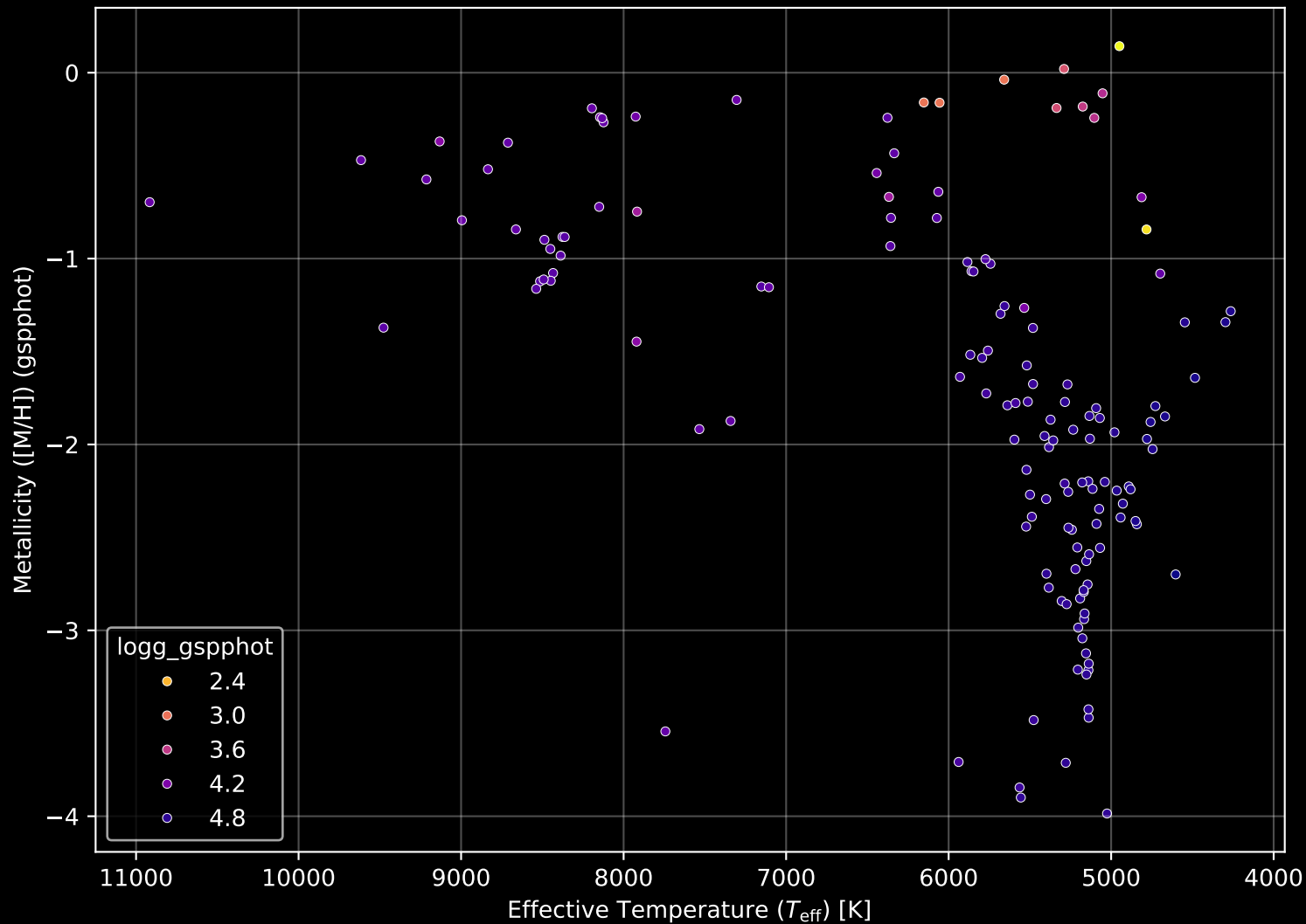
Gaia Cluster: [Dias_2] Stellar Population Parameters (n= 147)
