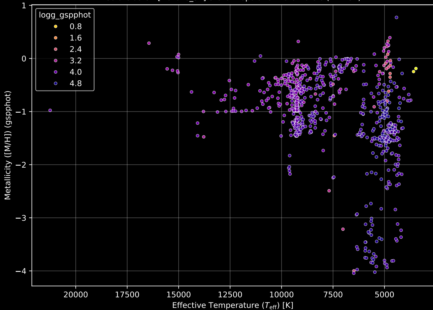
Gaia Cluster: [Dolidze_32] Stellar Population Parameters (n= 754)
