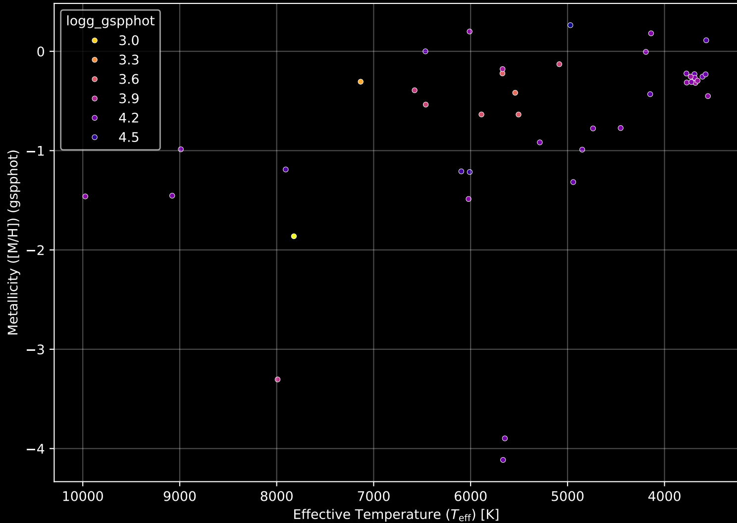
Gaia Cluster: [Dolidze_8] Stellar Population Parameters (n= 43)
