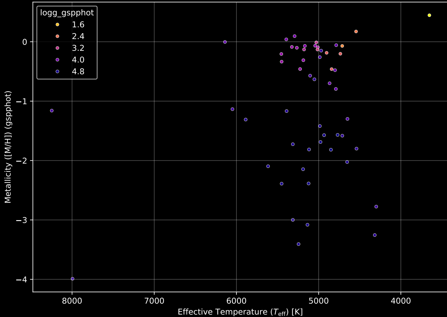
Gaia Cluster: [ESO_092_18] Stellar Population Parameters (n= 54)
