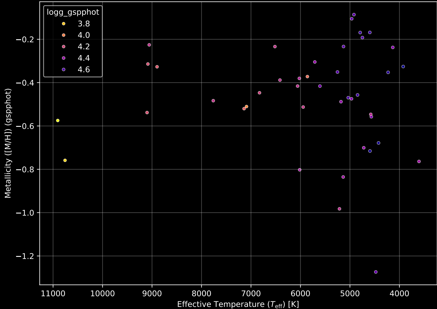
Gaia Cluster: [ESO_166_04] Stellar Population Parameters (n= 42)
