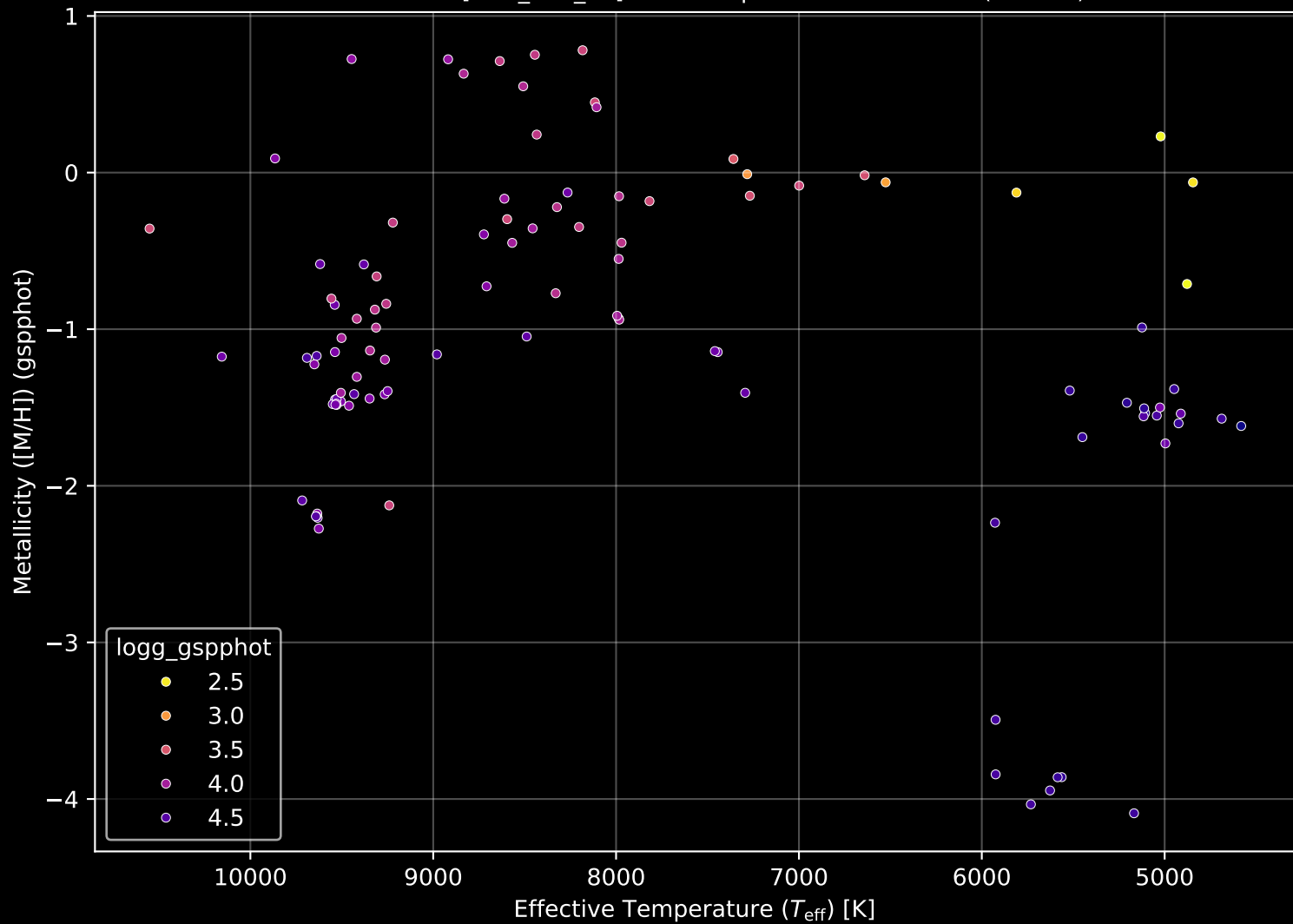
Gaia Cluster: [ESO_211_03] Stellar Population Parameters (n= 106)
