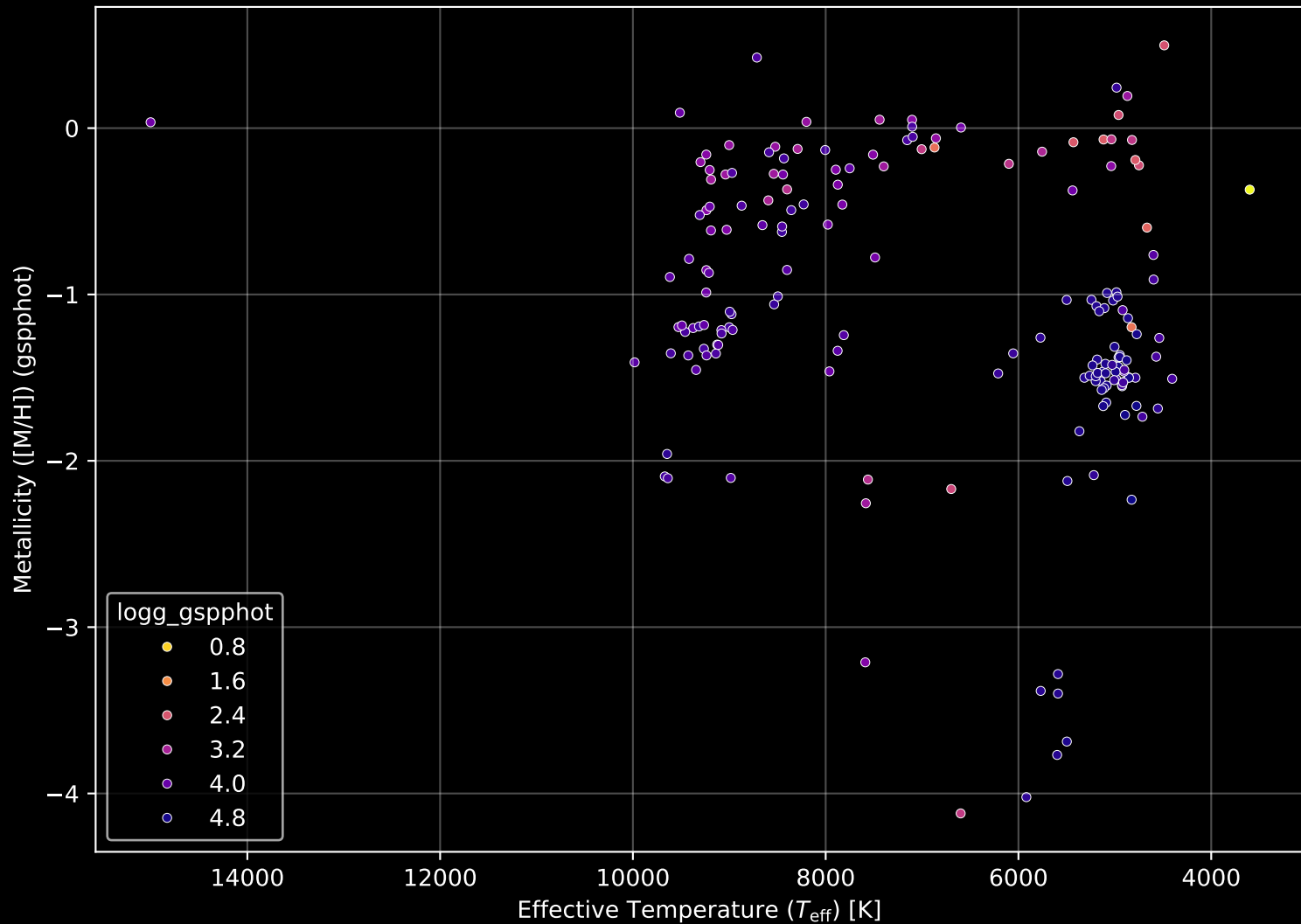
Gaia Cluster: [ESO_226_06] Stellar Population Parameters (n= 175)
