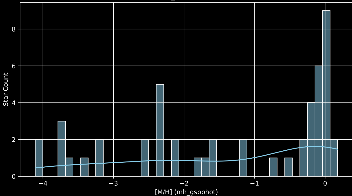
Gaia Cluster: [ESO_311_21 [M/H] (mh_gspphot) (n= 49)
