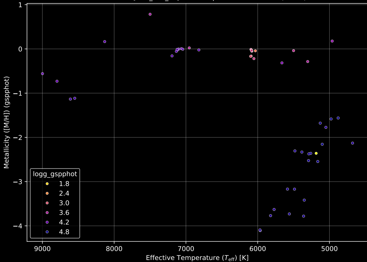
Gaia Cluster: [ESO_311_21] Stellar Population Parameters (n= 50)
