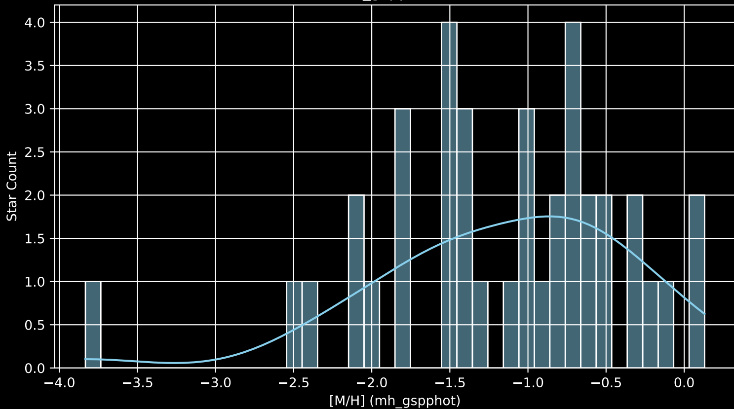
Gaia Cluster: [ESO_312_04 [M/H] (mh_gspphot) (n= 38)
