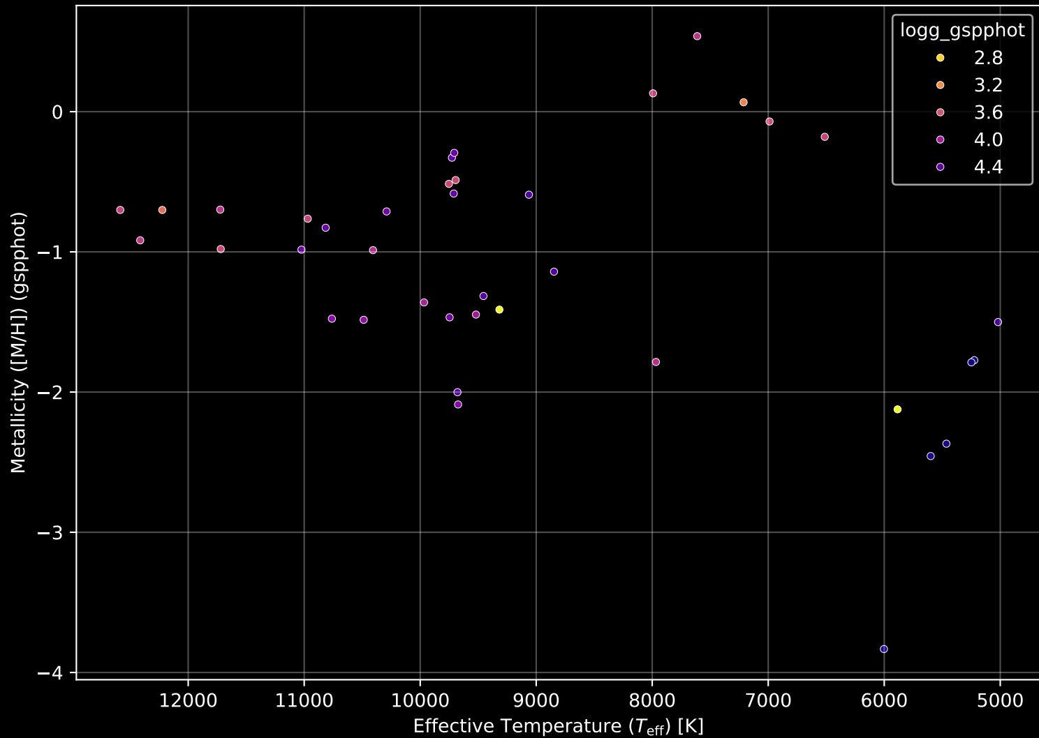
Gaia Cluster: [ESO_312_04] Stellar Population Parameters (n= 39)
