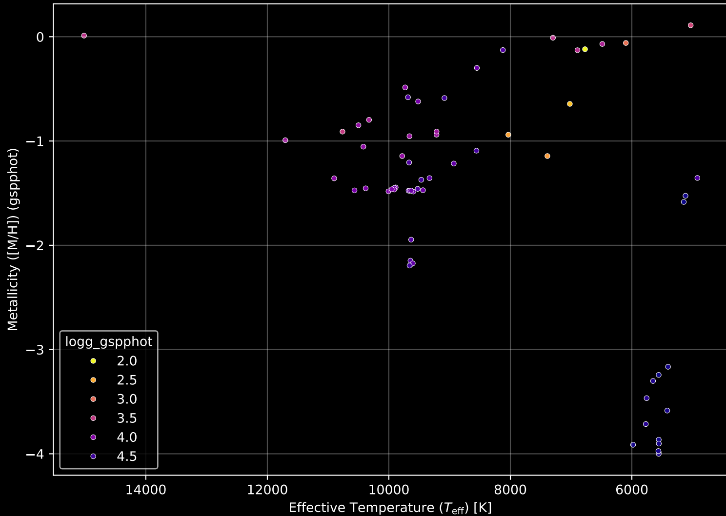
Gaia Cluster: [ESO_313_03] Stellar Population Parameters (n= 64)
