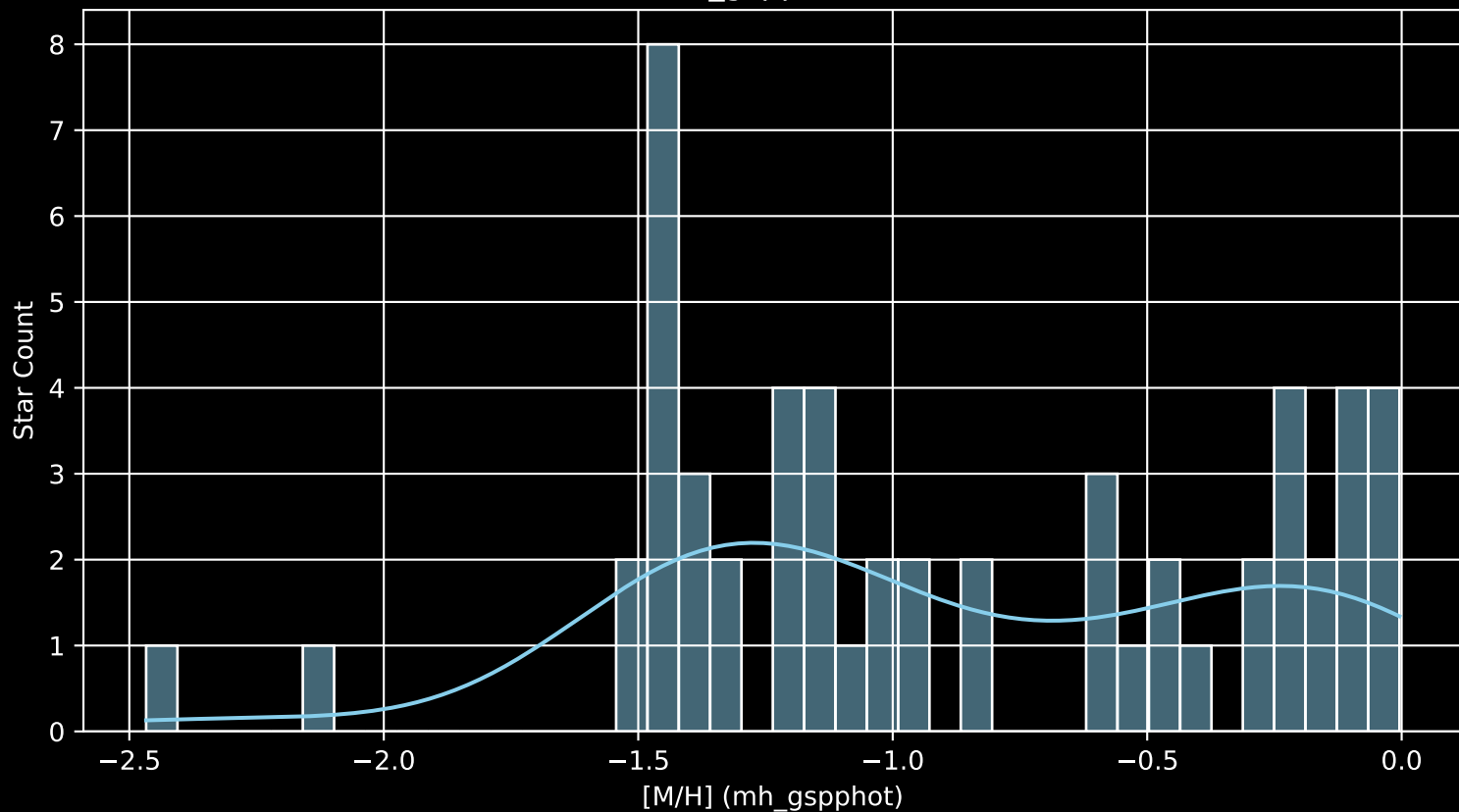
Gaia Cluster: [ESO_368_14 [M/H] (mh_gspphot) (n= 55)
