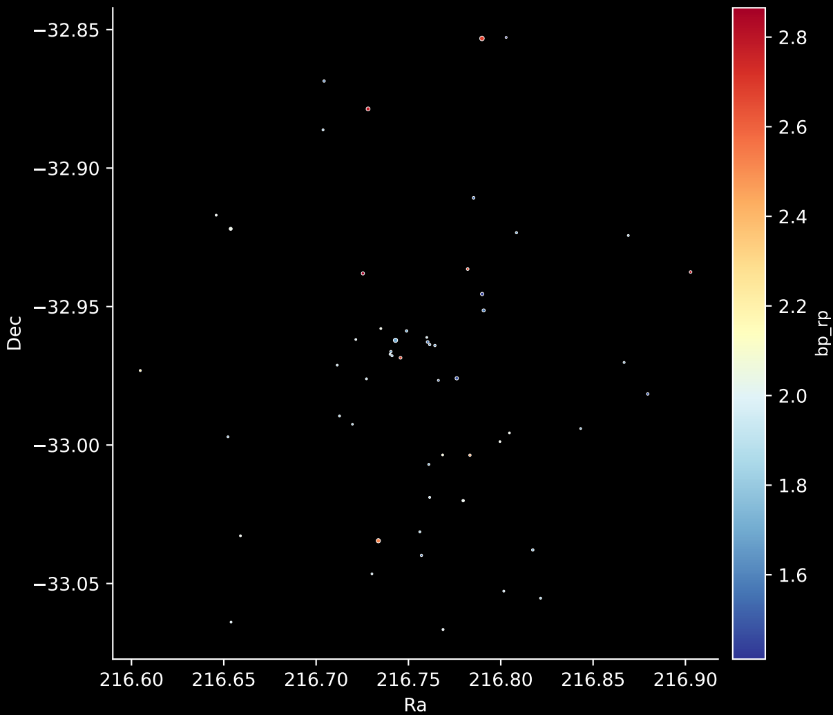
Gaia Cluster: [ESO_368_14] Stars: 55
