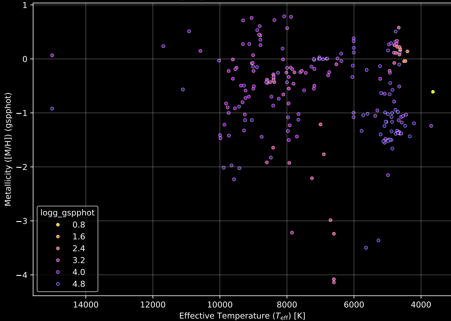
Gaia Cluster: [ESO_393_15] Stellar Population Parameters (n= 217)
