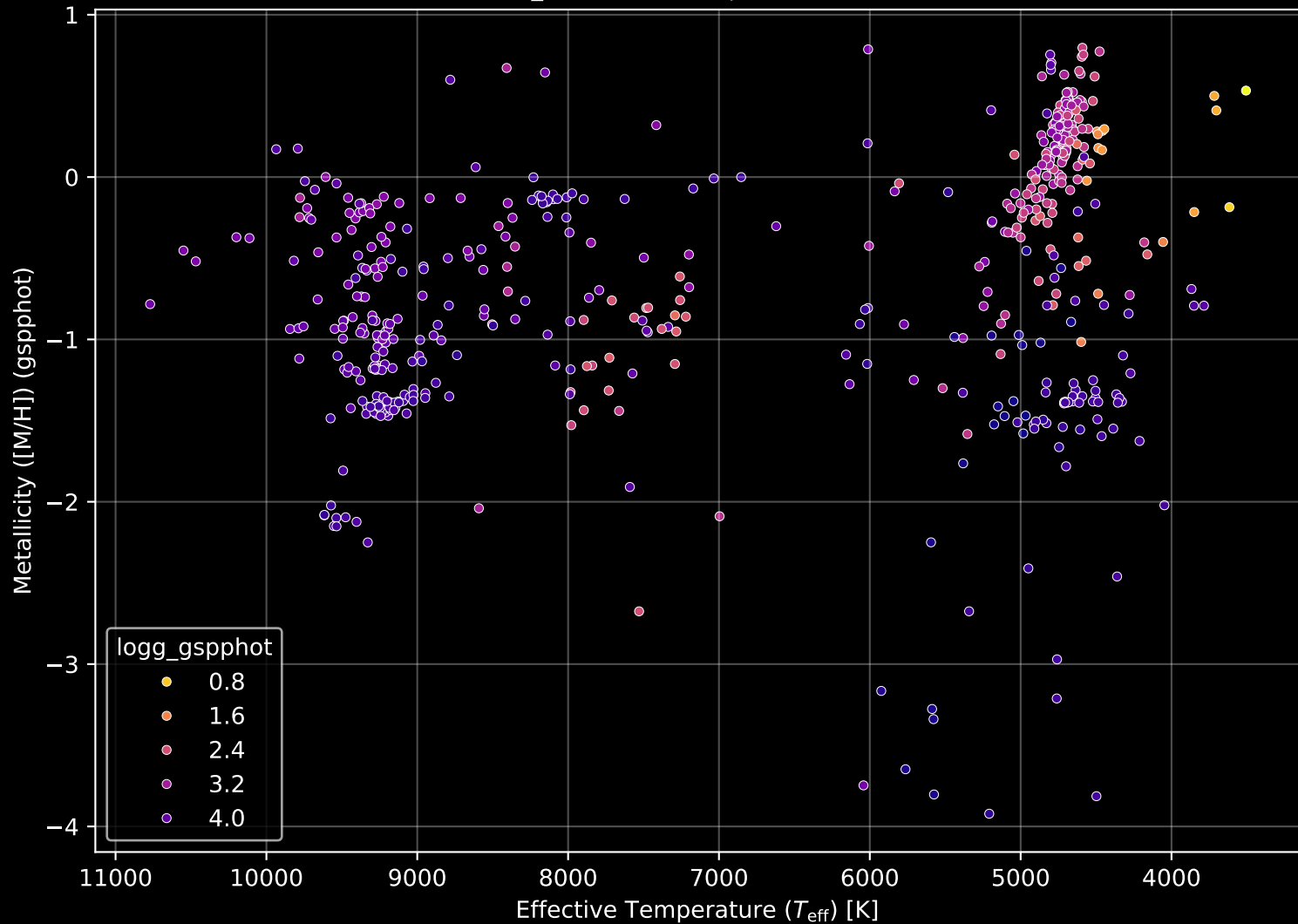
Gaia Cluster: [FSR_0088] Stellar Population Parameters (n= 540)
