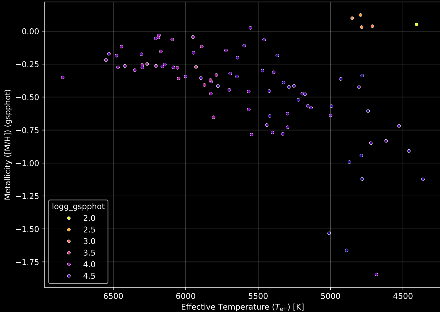
Gaia Cluster: [FSR_0278] Stellar Population Parameters (n= 87)
